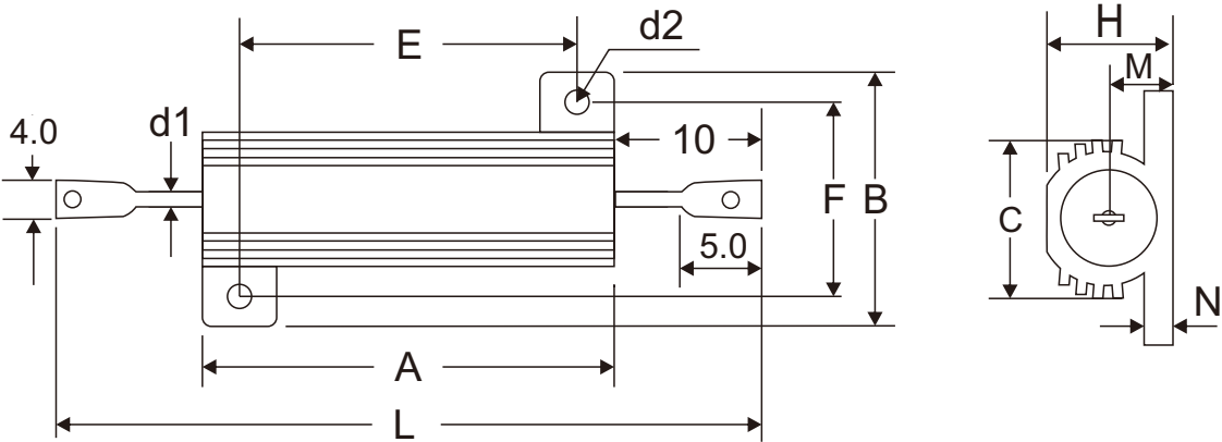
RXG24 5W-50W外形及产品尺寸
